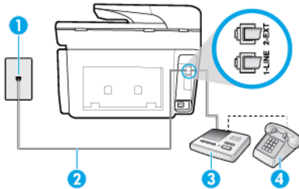
Afbeelding 5-11 Achteraanzicht van de printer
