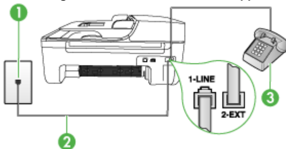
Afbeelding 7-4 Achteraanzicht van het apparaat
