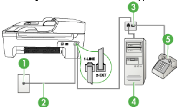
Afbeelding 7-8 Achteraanzicht van het apparaat
